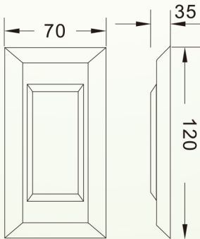
正視圖
