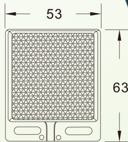
正視圖
