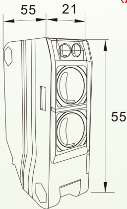
正視圖
